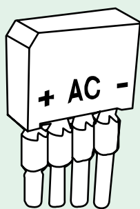
4603 RECTIFIER
